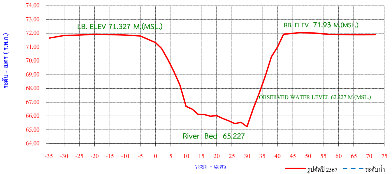
รูปตัดขวางลำน้ำ ปีน้ำ 2567 สถานี P.78 คลองขลุ้ง อ.คลองขลุ้ง จ.กำแพงเพชร
